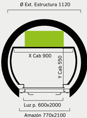
RUND Mindest-Schachtkopf 2600m
