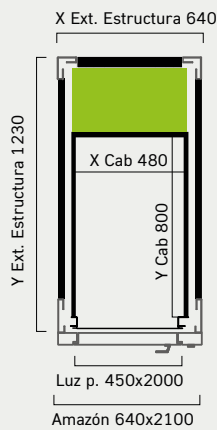
OHNE TÜREN Mindest-Schachtkopf 2600m
